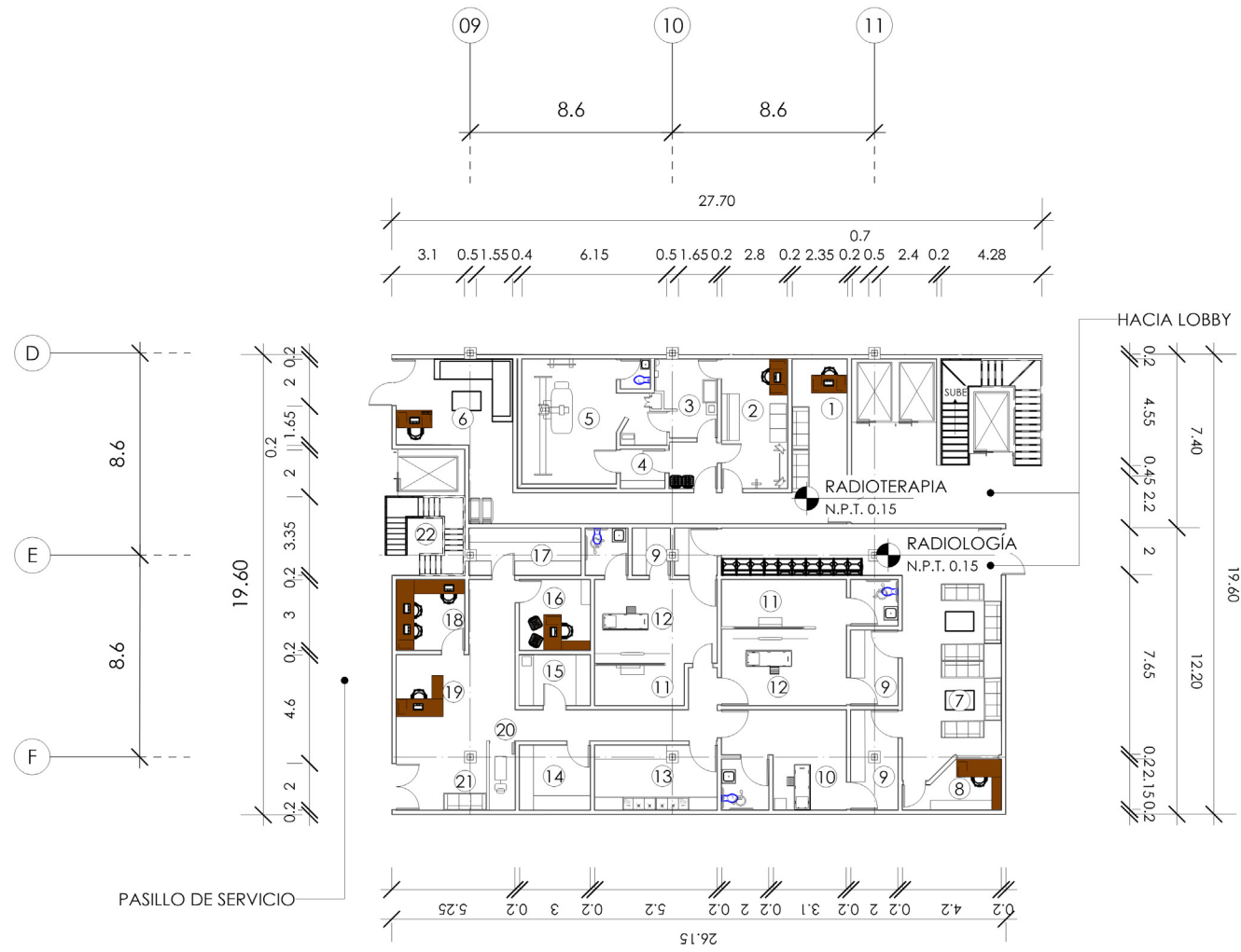
① RADIOLOGÍA Y RADIOTERAPIA 1:300
