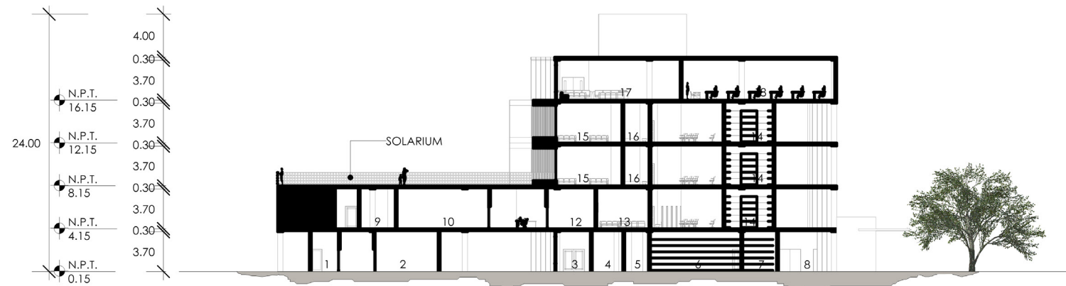
2 SECCIÓN B-B' 1:500
