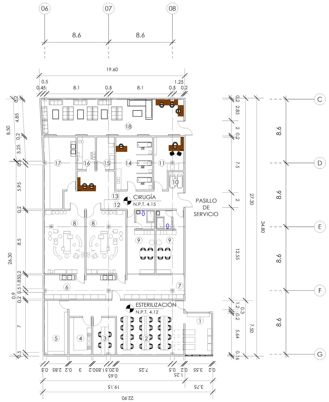
1 ESTERILIZACIÓN Y CIRUGÍA 1:300
