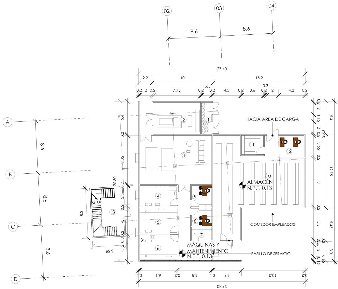
① ALMACÉN, MÁQUINAS Y MANTENIMIENTO 1:300
