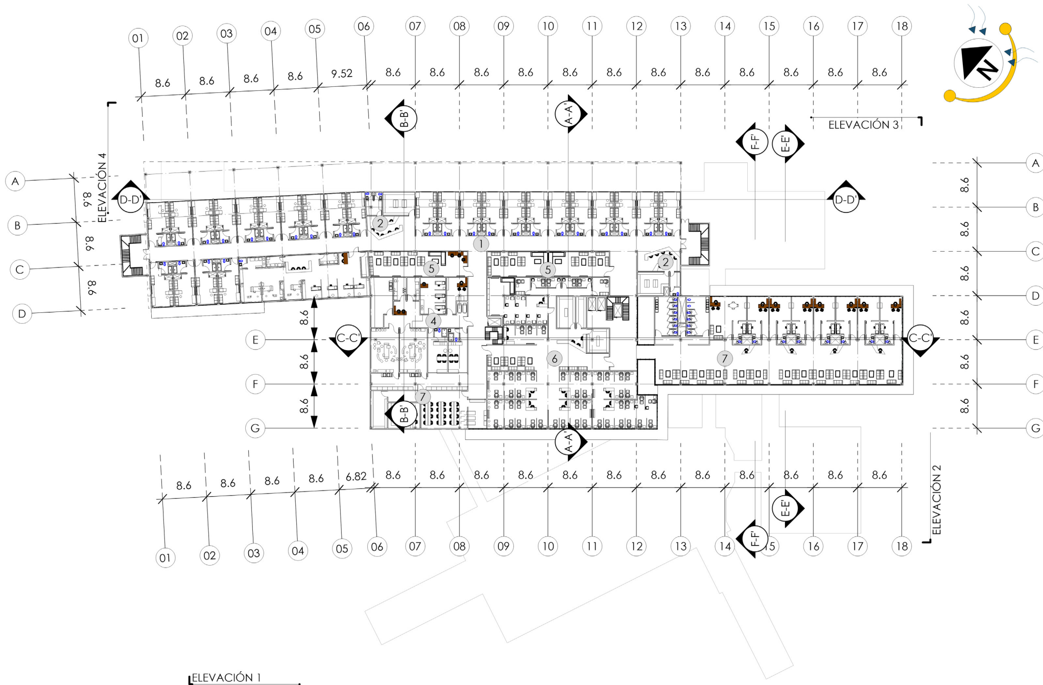
01 PLANTA ARQUITECTÓNICA N-02 1:750
