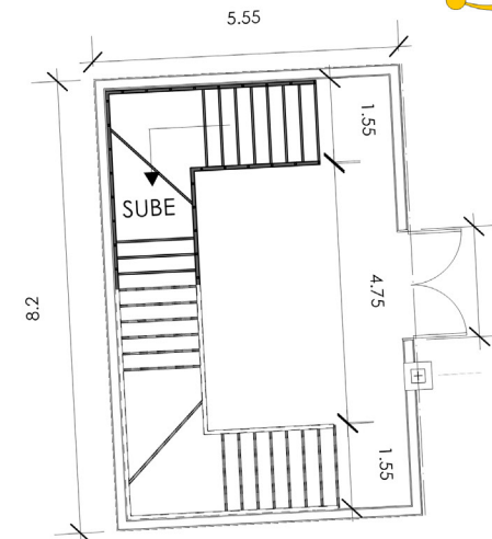
② ESCALERA DE EMERGENCIA 1:150
