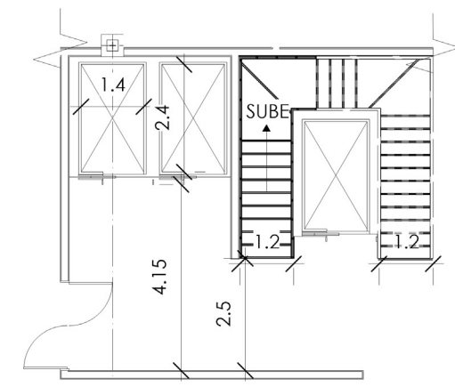
② ACCESO VERTICAL 1:150
