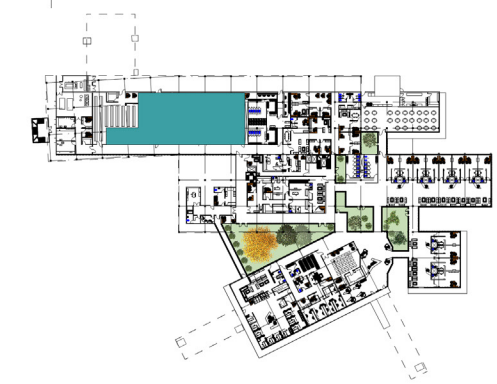
1 COCINA Y LAVANDERÍA 1:300
