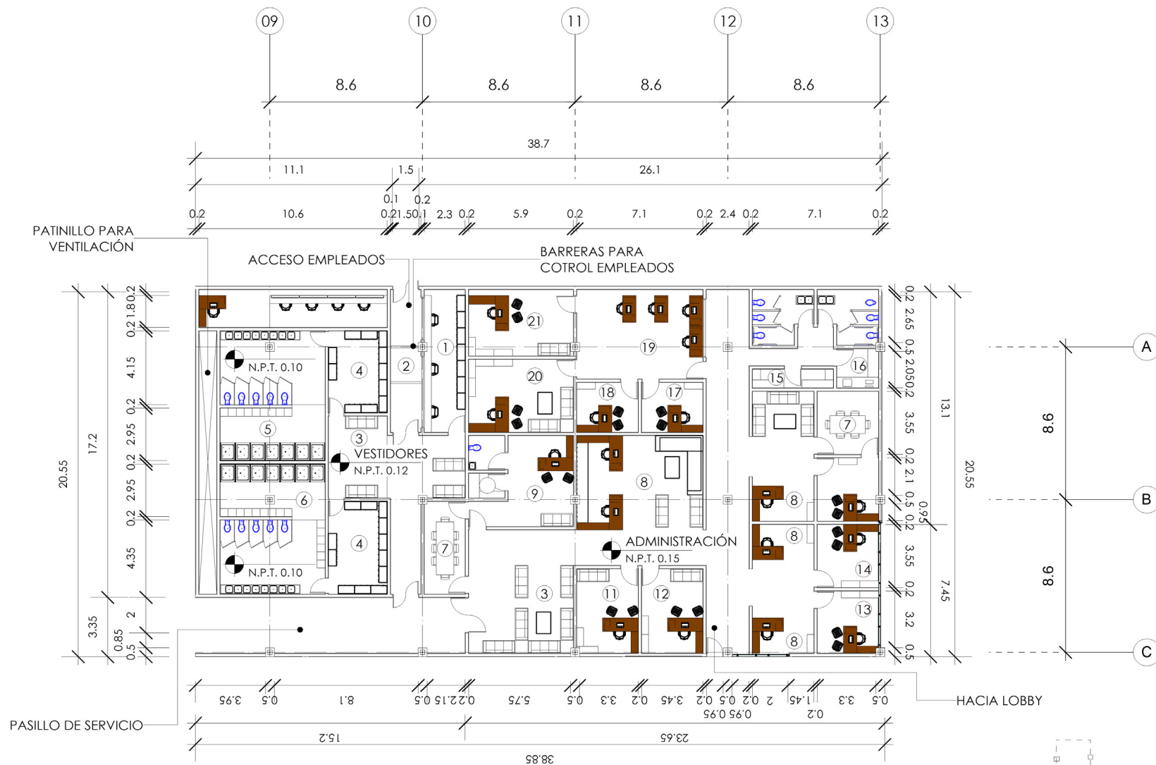
1 ADMINISTRACIÓN Y VESTIDORES 1:300
