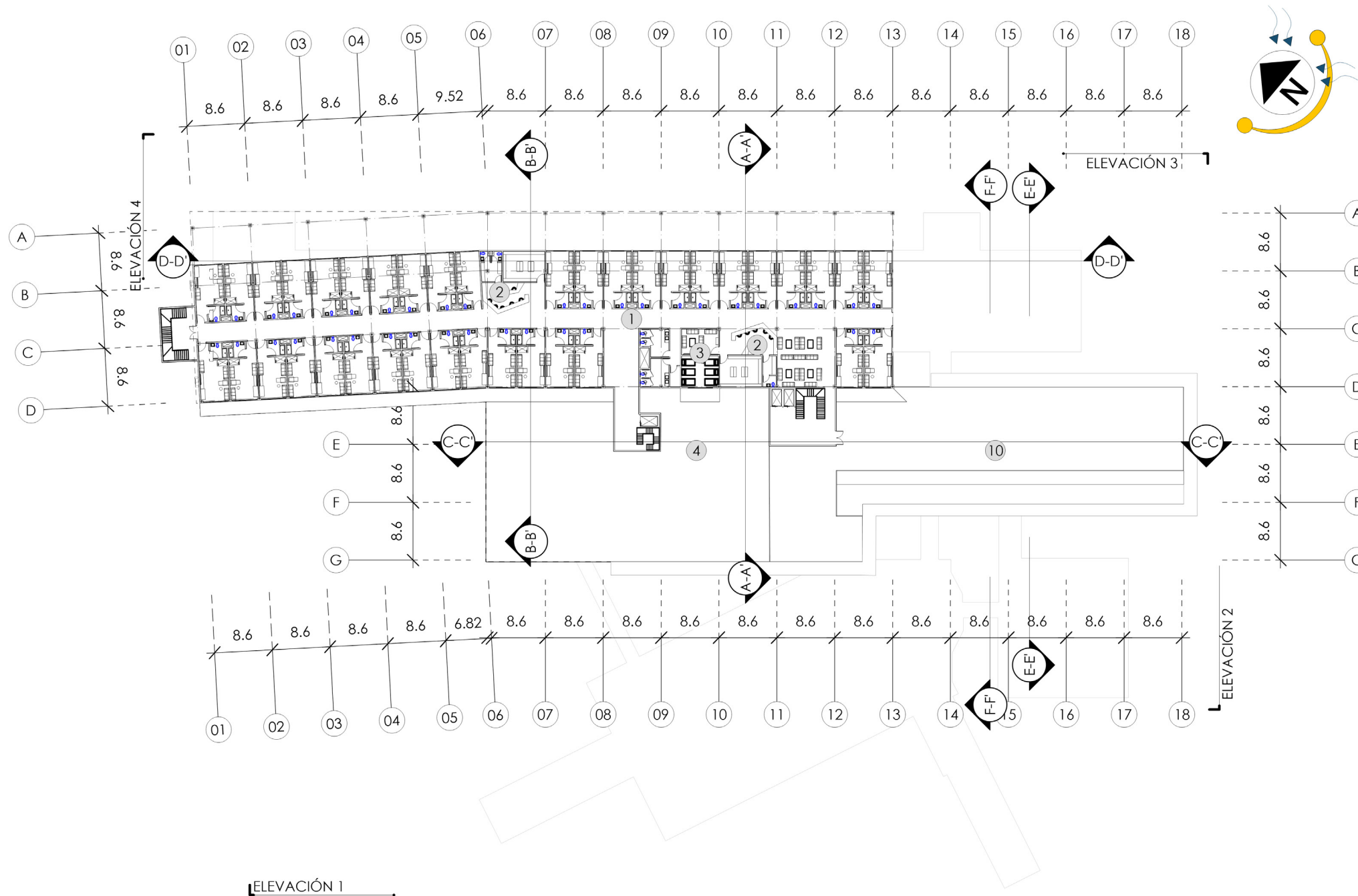
01 PLANTA ARQUITECTÓNICA N-03 1:750
